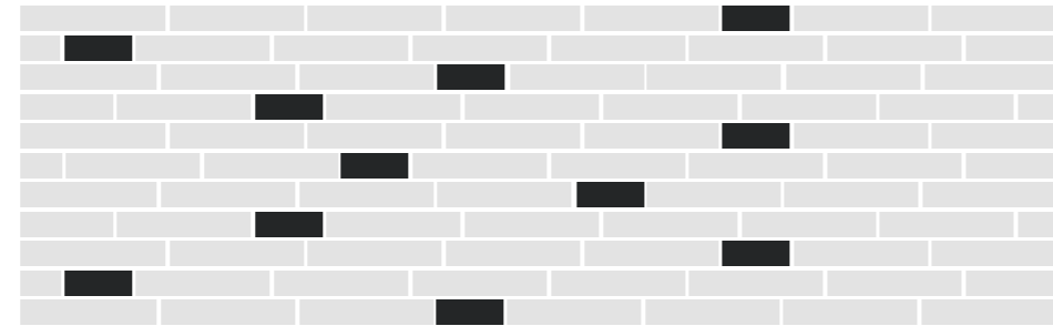
Wilder Verband
