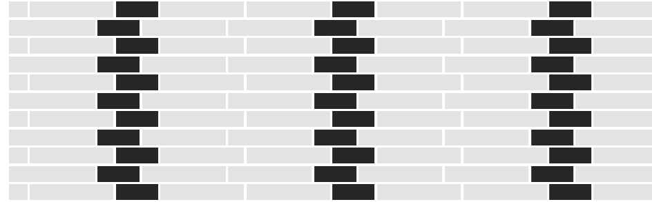
Schlesischer Verband
